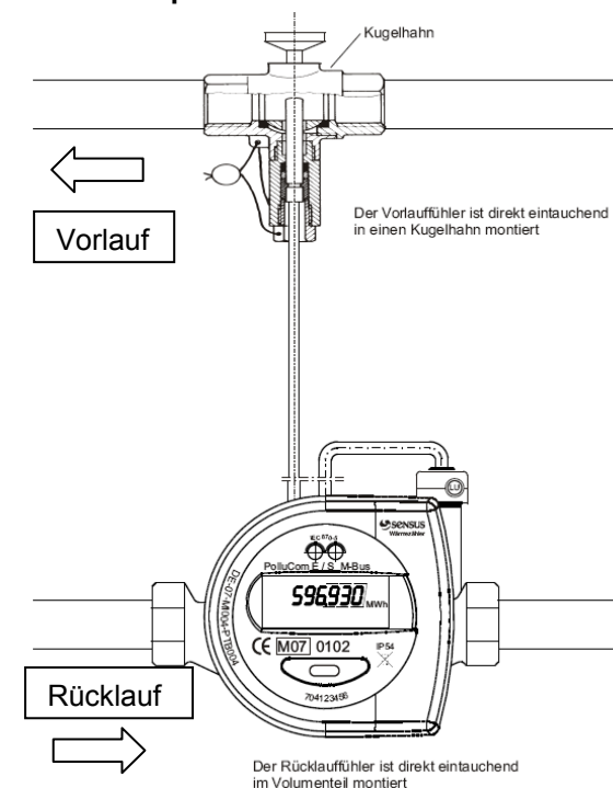
Abb. 1: Einbau im Rücklauf einer Heizungsanlage, Vorlauftemperaturfühlereinbau in Kugelhahn
