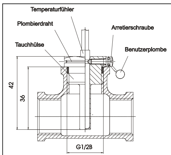
Abb. 2: Einbaubeispiel in T-Stück
